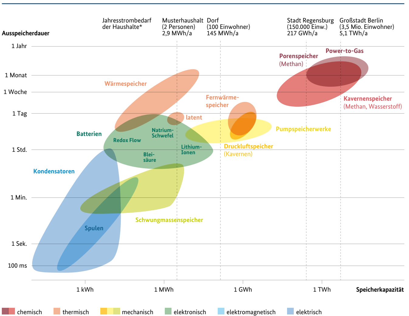
Abb. 10: Energiespeicher nach Ausspeicherdauer und Speicherkapazität
